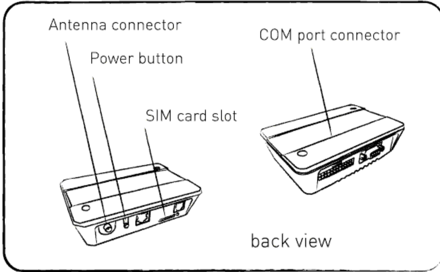
1x Siemens TC-65 modem
